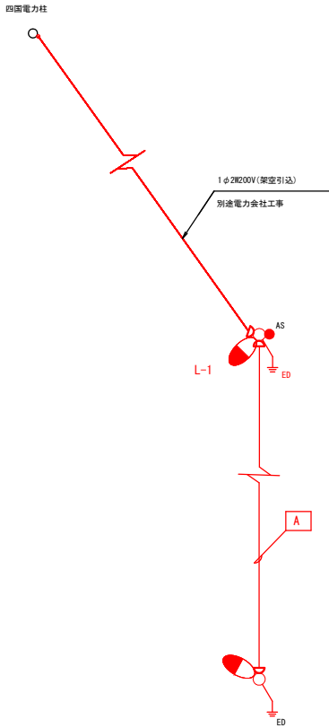
系 統 図
